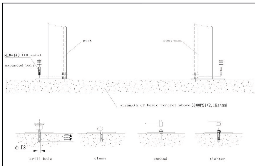
Figure 3 (installation des deux colonnes)
