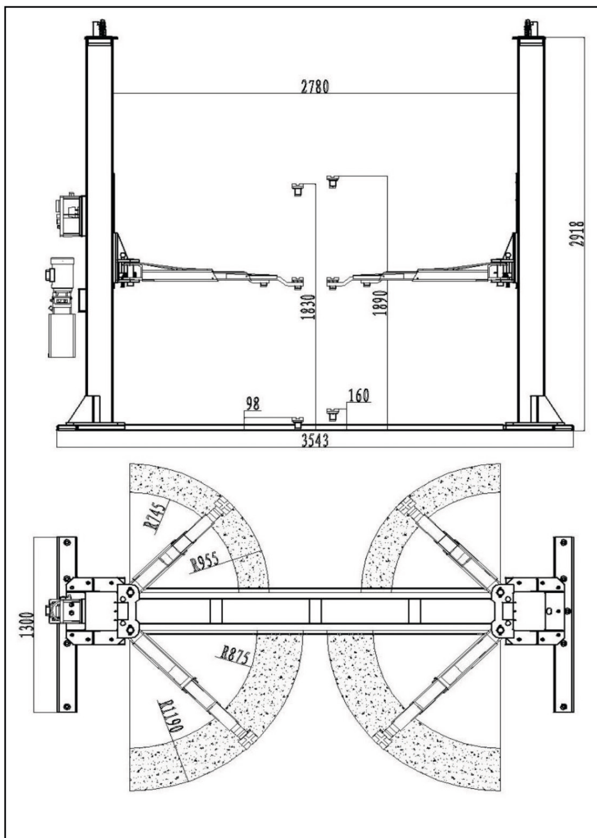
Figure 1 (Dimensions de le pont élévateur)
